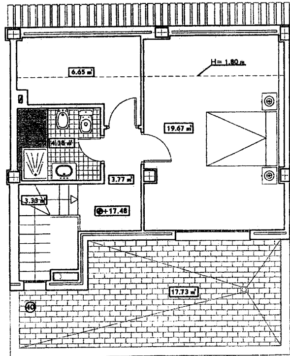
PLANTA ALTA
